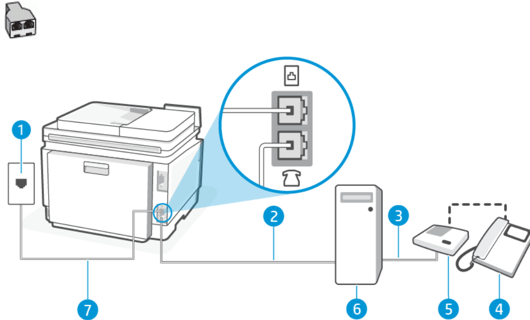
Abbildung 7-4 Beispiel für einen Splitter für parallele Leitungen
